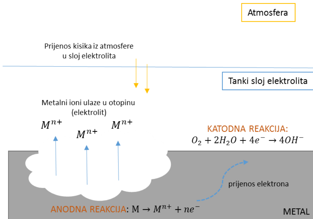
Slika 1. Mehanizam atmosfere korozije. 4
