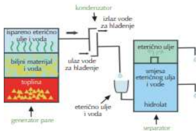
Slika 2. Shematski prikaz postupka vodene destilacije
