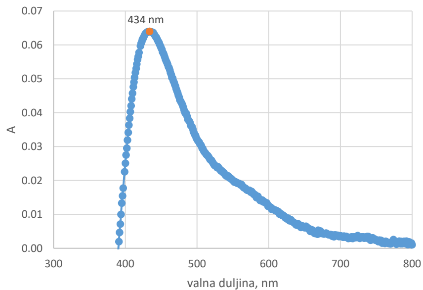
Slika 19. Apсорpcijski spektar koloidnog srebra dobiven pri pH = 7
