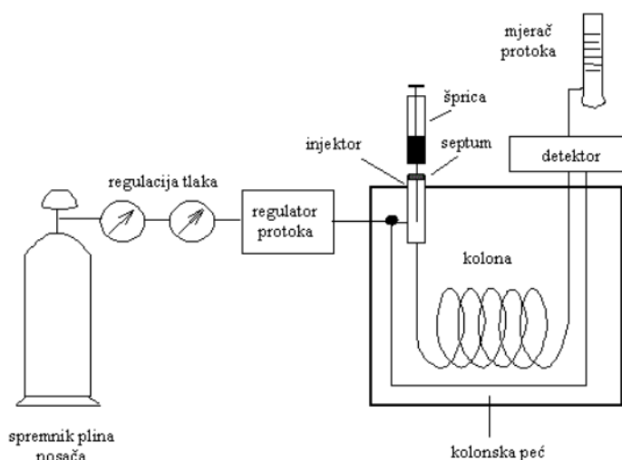
Slika 7. Shematski prikaz plinskog kromatografa 19
