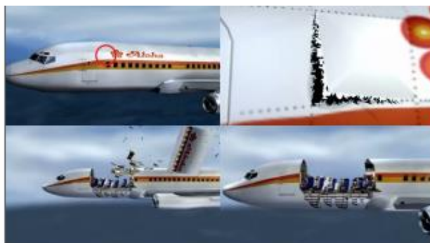
Slika 29. Simulacija leta aviona Boeing 737, Aloha Airlines, let 243. 19,21
