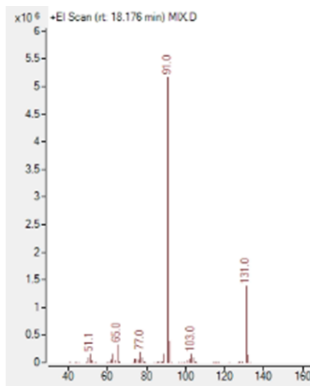
Slika 19. Spektar masa 3-fenilpropanonitrila
