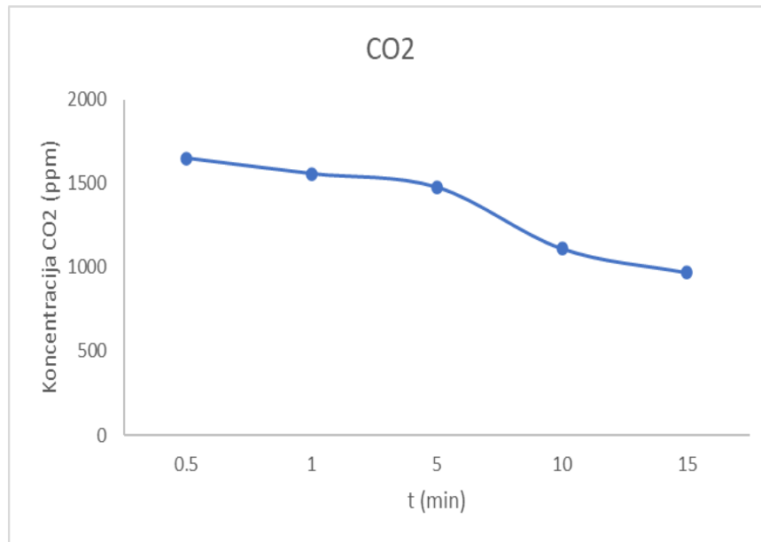
Slika 15. Grafički prikaz promjene koncentracije CO 2 s vremenom.
