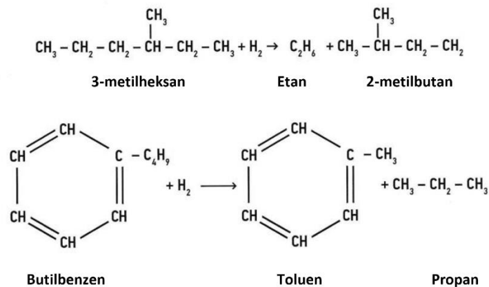
Slika 5. Reakcije hidrokrekiranja 2
