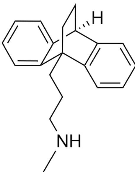
Slika. 15. Struktura maprotilina
