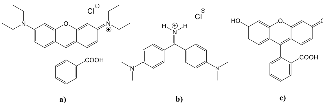
Slika 11. Kemijske strukture istraživanih fluorescentnih boja:
