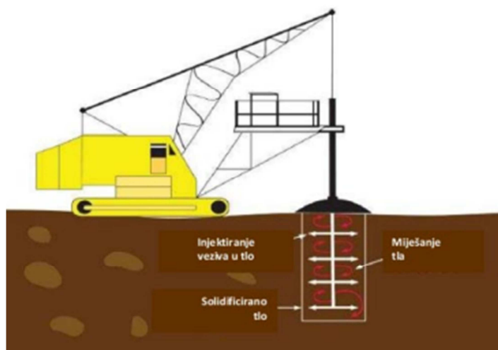
Slika 1.15. Shema stabilizacije/solidifikacije 29
