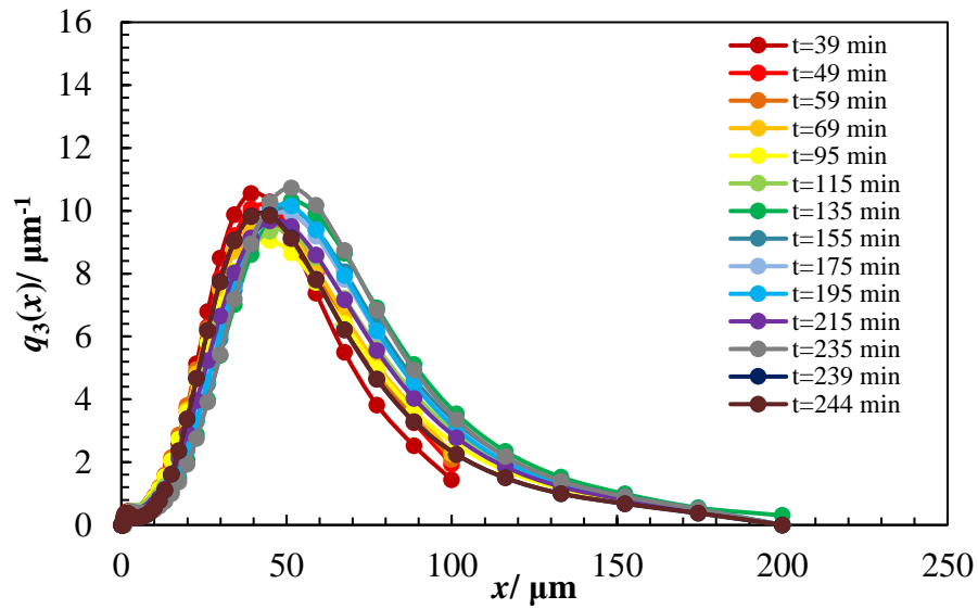
Slika 17. Funkcije gustoće raspodjele kristala tijekom sonokristalizacije pri brzini hlađenja matične otopine od 4\text{ }^\circ\text{C h}^{-1} ( N_{\text{JS}} = 324\text{ o min}^{-1} , A = 20\% , T_z = 30\text{ }^\circ\text{C} ).
