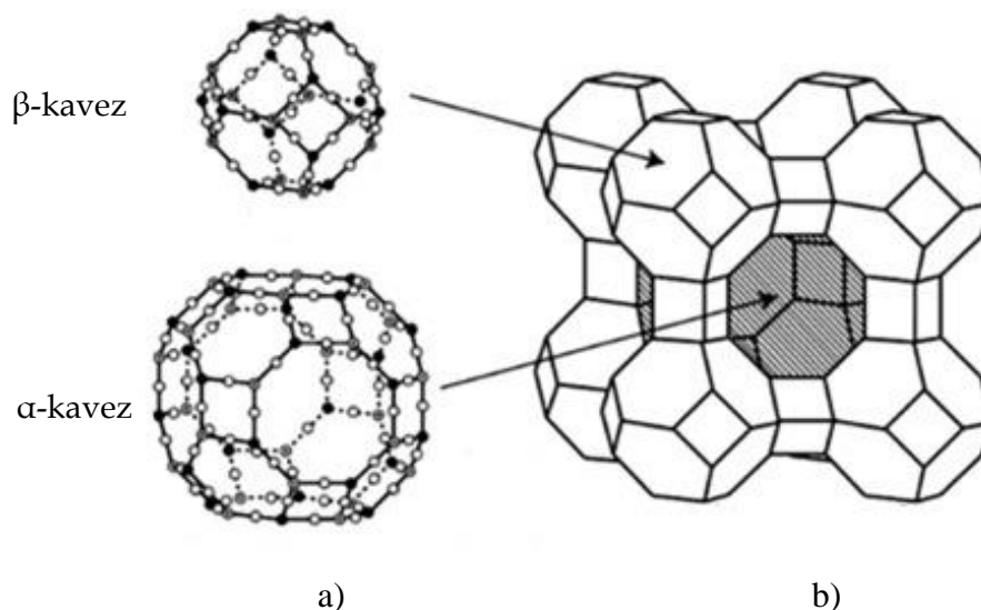
Slika 1.4. a) Tercijarne strukture zeolita; b) Prostorna mrežna struktura zeolita. 26
