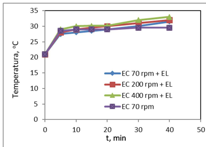
Slika 4. 5. Promjena temperature u ovisnosti o vremenu t za uzorke bez dodatka zeolita pri različitim brzinama vrtnje miješala
