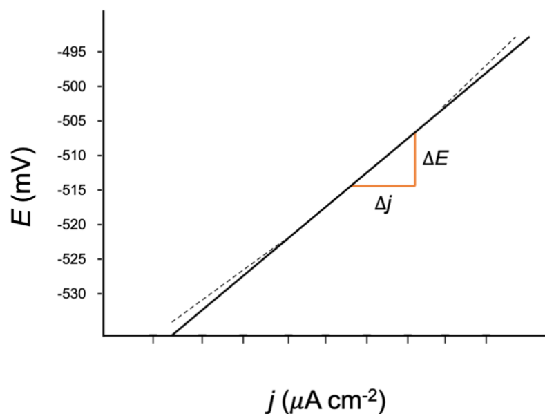
Slika 28. Određivanje polarizacijskog otpora iz nagiba polarizacijske krivulje u blizini korozivnog potencijala.
