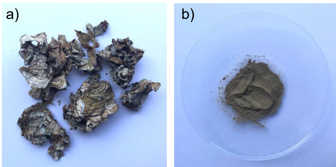
Slika 30. Uzorak Padina pavonica : a) osušeni, b) homogenizirani.
