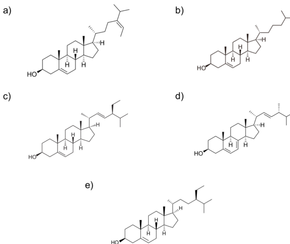
Slika 22. Kemijska struktura nekih sterola prisutnih u smeđim algama: a) fukosterola, 204 b) kolesterola, 205 c) stigmasterola, 206 d) ergosterola, 207 e) \beta -sitosterola. 208
